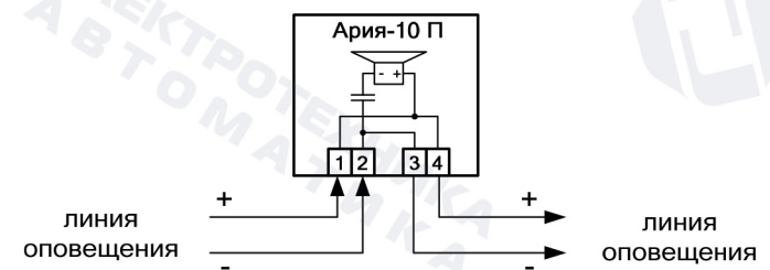
Рис.1. Схема подключения.
