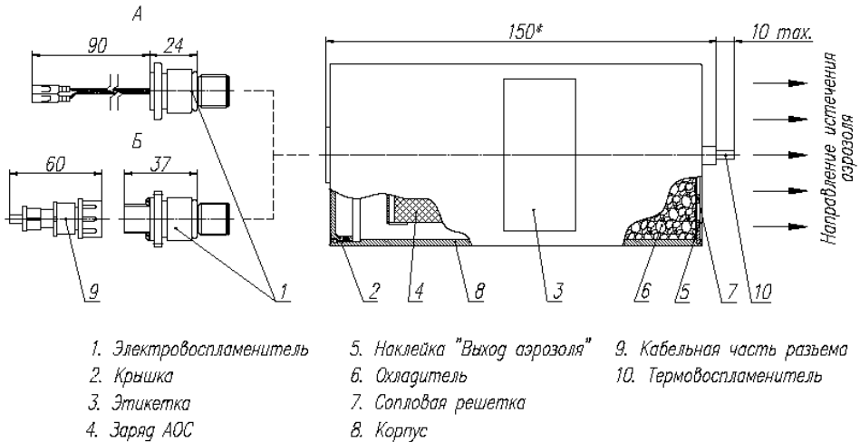
Рис.1. Генератор огнетушащего аэрозоля.
